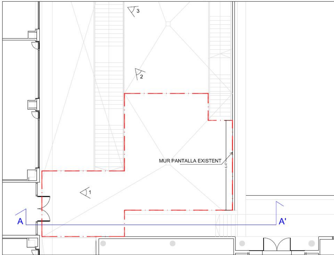
PLÀNOL PLANTA UBICACIÓ PATI ZONA ACTUACIÓ
